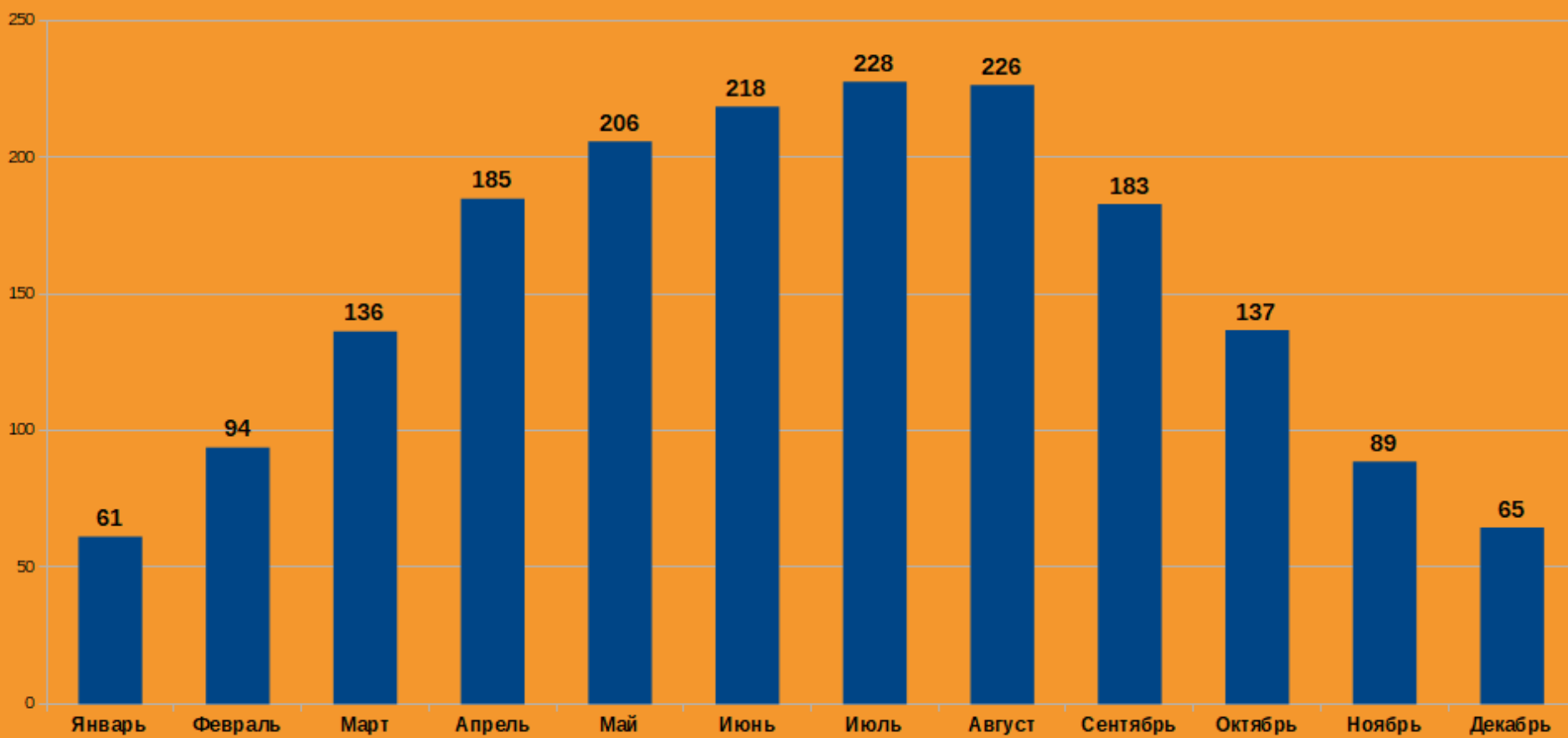
Ежемесячная выработка энергии МВт/ч в месяц
